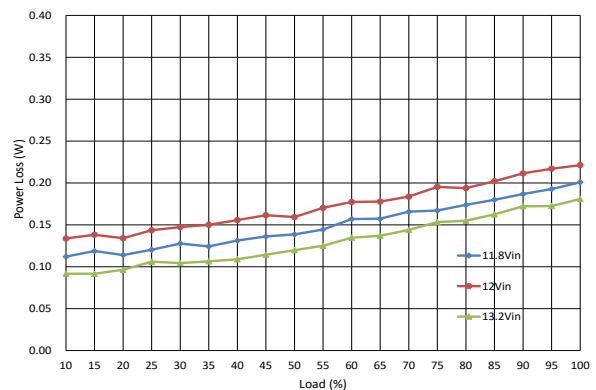
EVP1F12S05 Module
